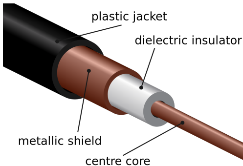
Abbildung: Koaxialkabel, Tkgd2007 2008, cc by, Coaxial_cable_cutaway.svg
