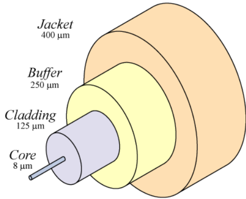
Abbildung: Singlemode_fibre_structure.png cc by-sa DrBob , Wikipedia
