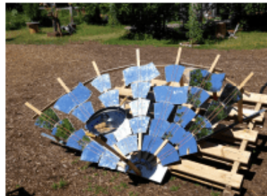
Selbstbau-Parabolspiegel gebrauchte Spiegel 1.5m² (15 €), Glasschneider (10 €), gebrauchter Lattenrost 140 cm (20 €), mit Kleinkram insgesamt ca. 50 €
